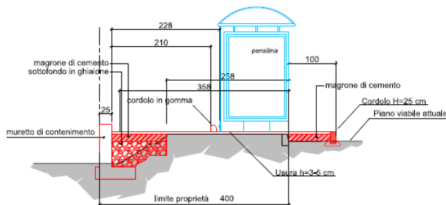
stato attuale - 1:50
