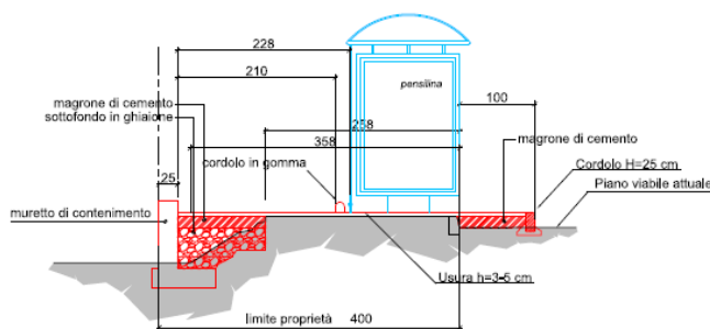
stato attuale - 1:50
