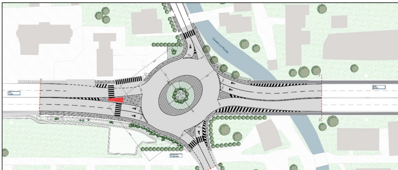
Figura 3 Stralcio planimetria di progetto selezionata
