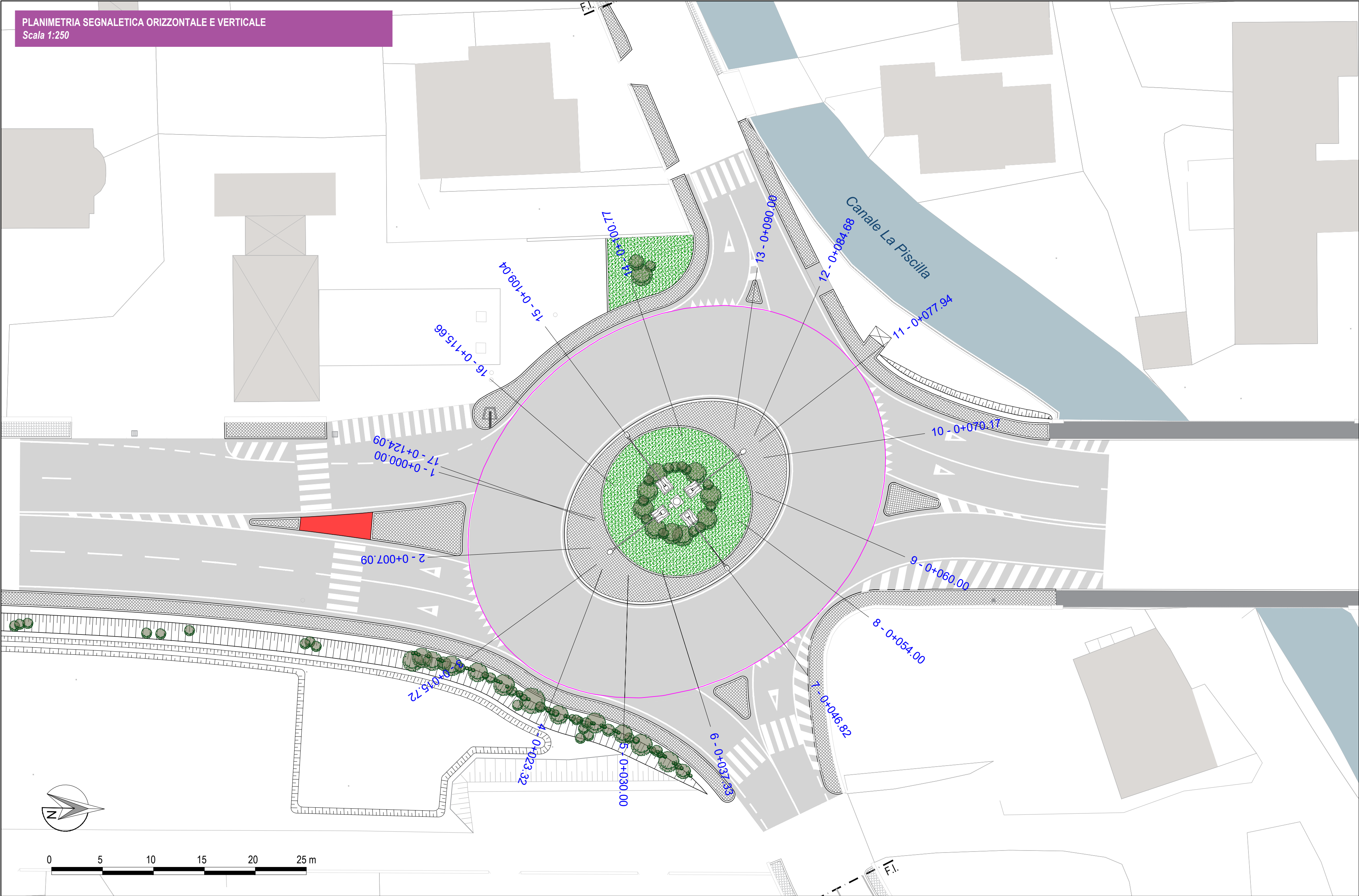
PLANIMETRIA DI PROGETTO CON TRACCIA DELLE SEZIONI TRASVERSALI Scala 1:250
