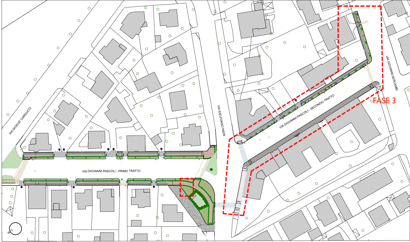
LAYOUT DI CANTIERE - FASE 3
