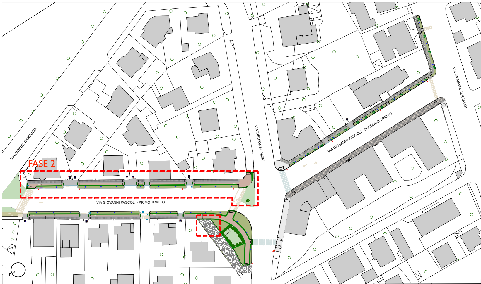
LAYOUT DI CANTIERE - FASE 2
