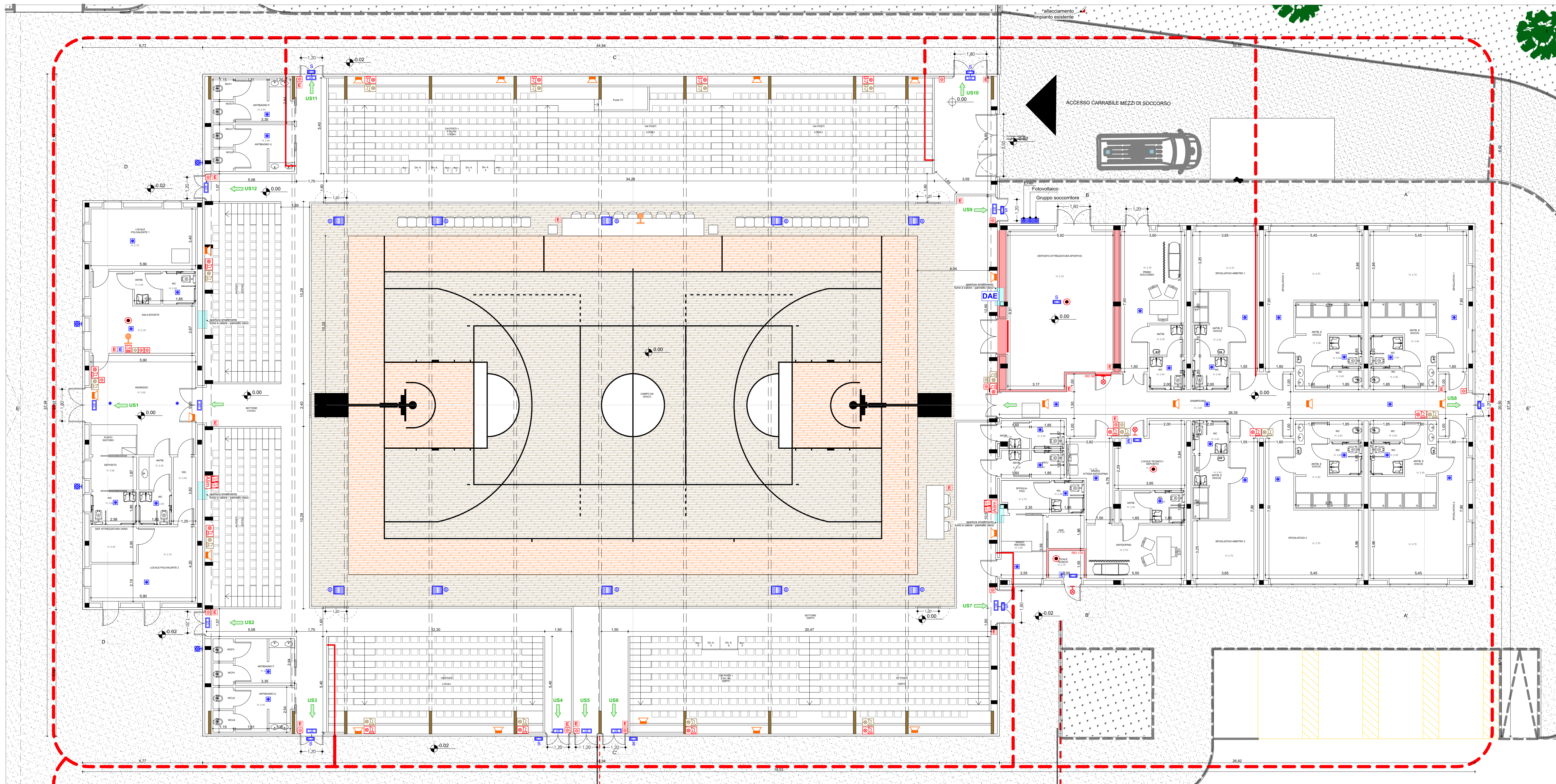
1:100
