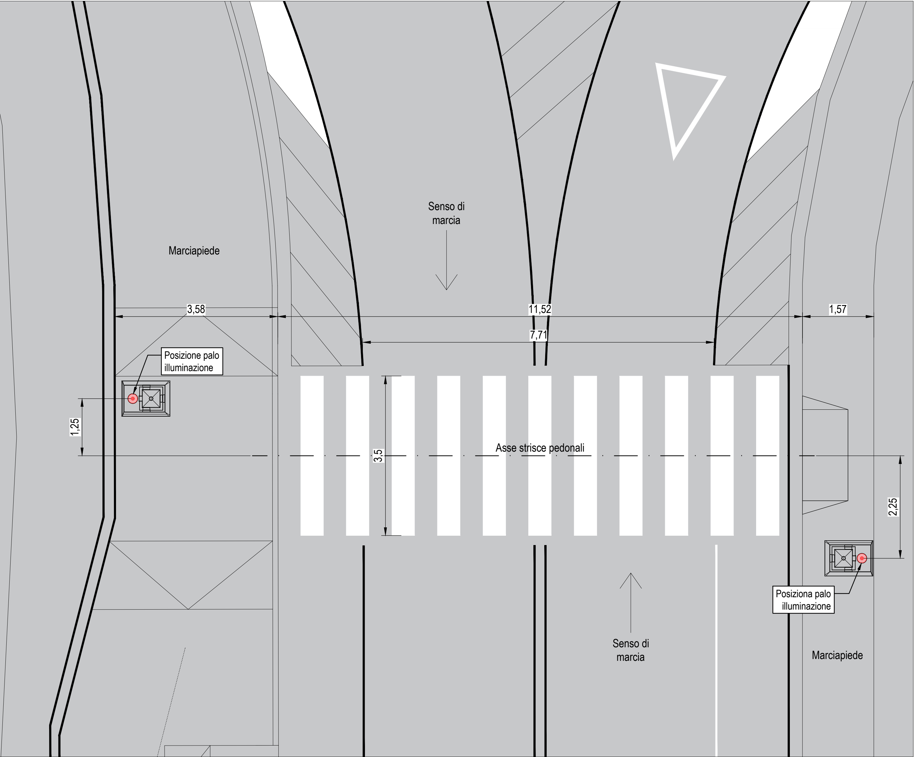
ATTRAVERSAMENTO PEDONALE 2 Particolare posizionamento palo illuminazione SCALA 1:50
