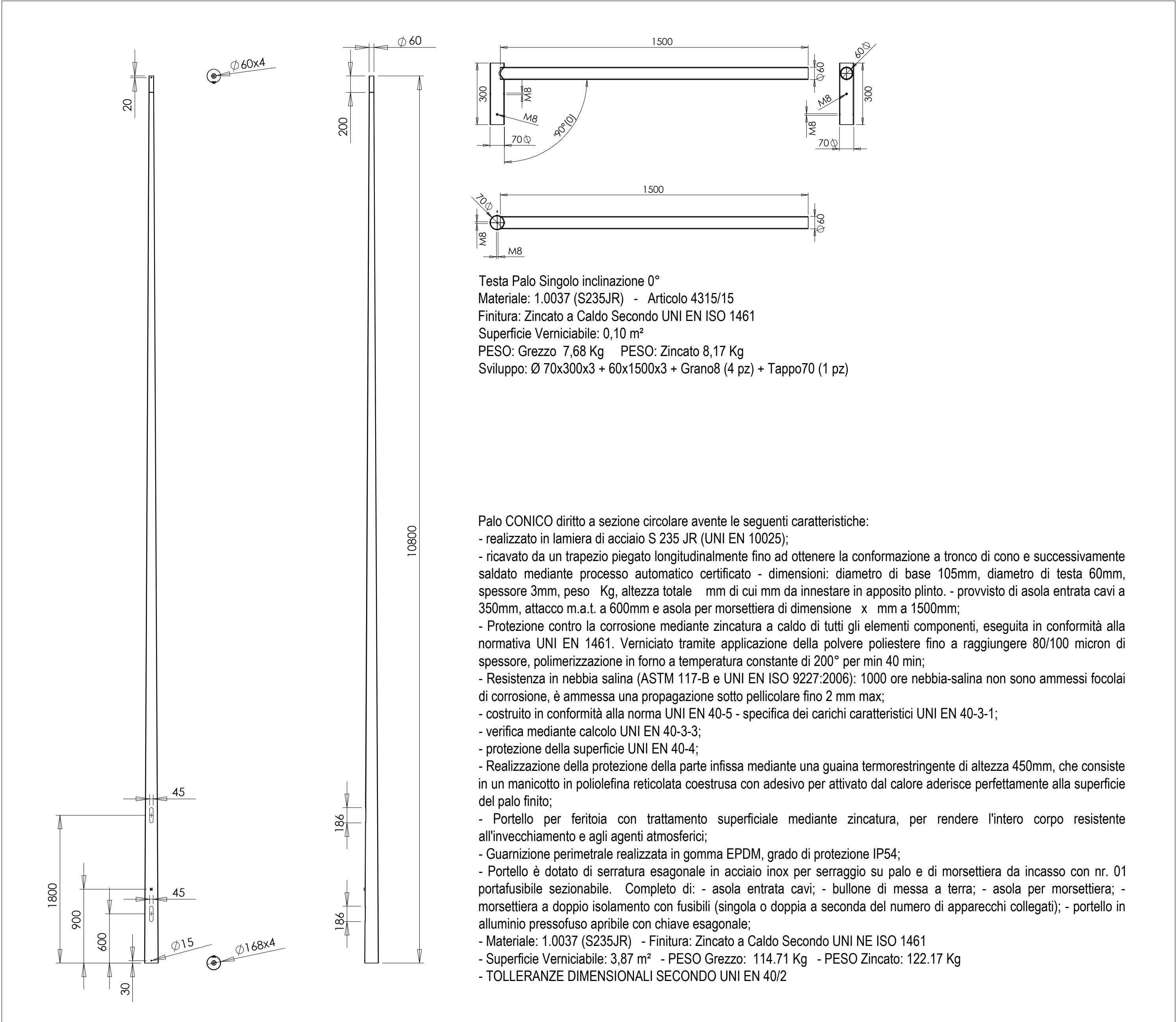
PALO CONICO DRITTO Caratteristiche dimensionali FUORI SCALA
