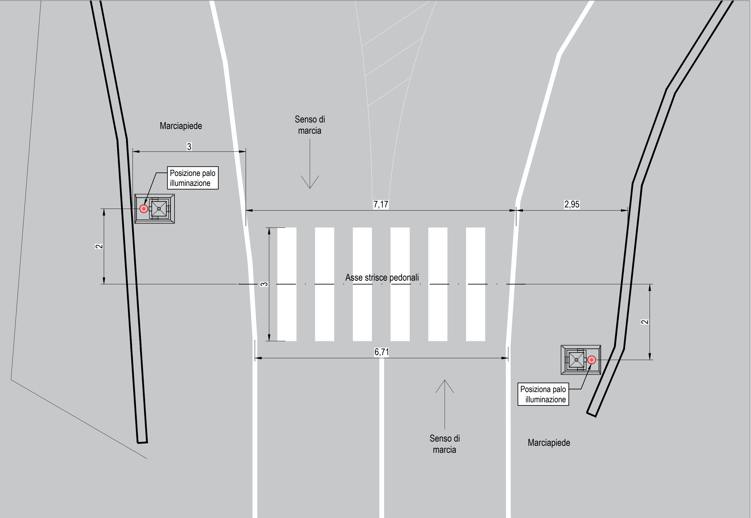
ATTRAVERSAMENTO PEDONALE 1 Particolare posizionamento palo illuminazione SCALA 1:50
