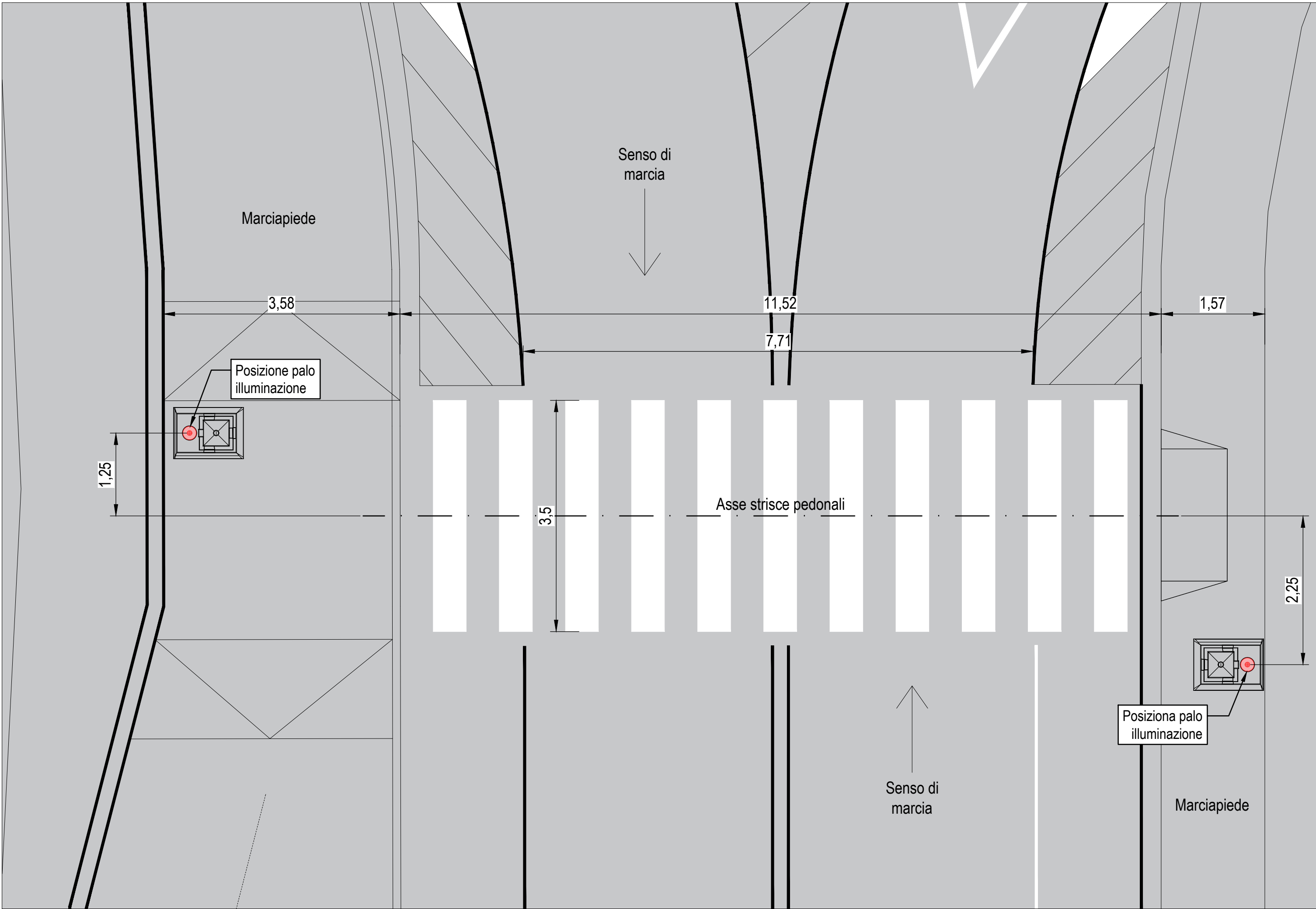
ATTRAVERSAMENTO PEDONALE 3 Particolare posizionamento palo illuminazione SCALA 1:50
