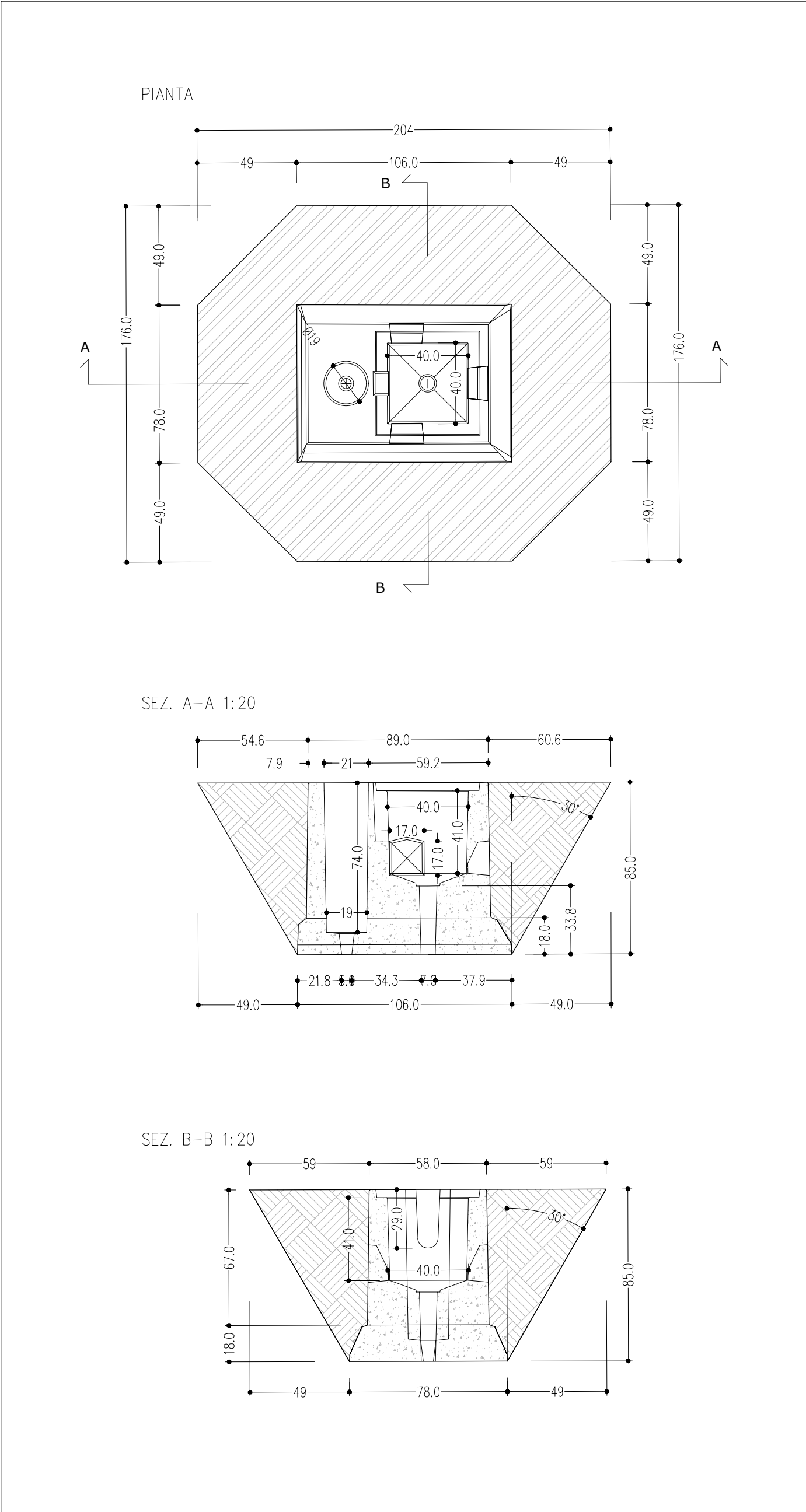
PLINTO DI FONDAZIONE PREFABBRICATO Caratteristiche dimensionali FUORI SCALA
