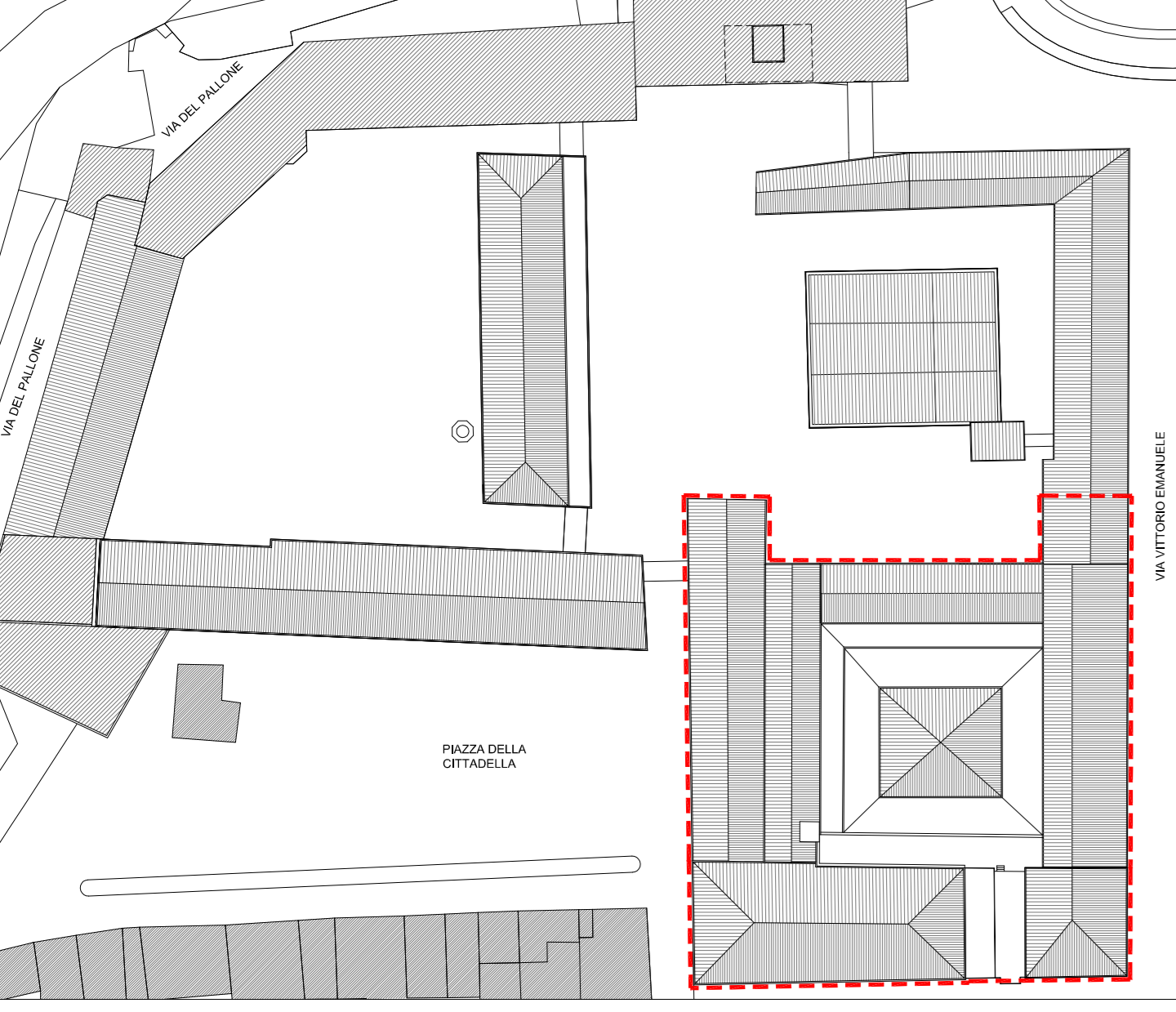
PLANIMETRIA GENERALE_SCALA 1:1.000
