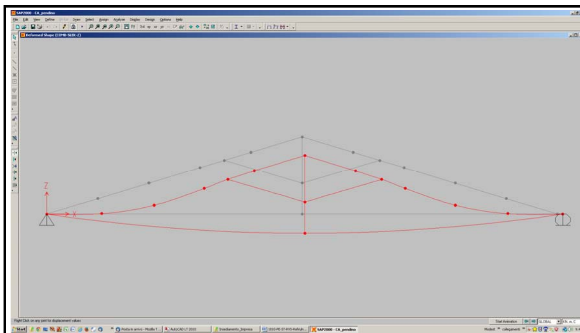
Fig. 37– Deformata elastica-SLER-2
