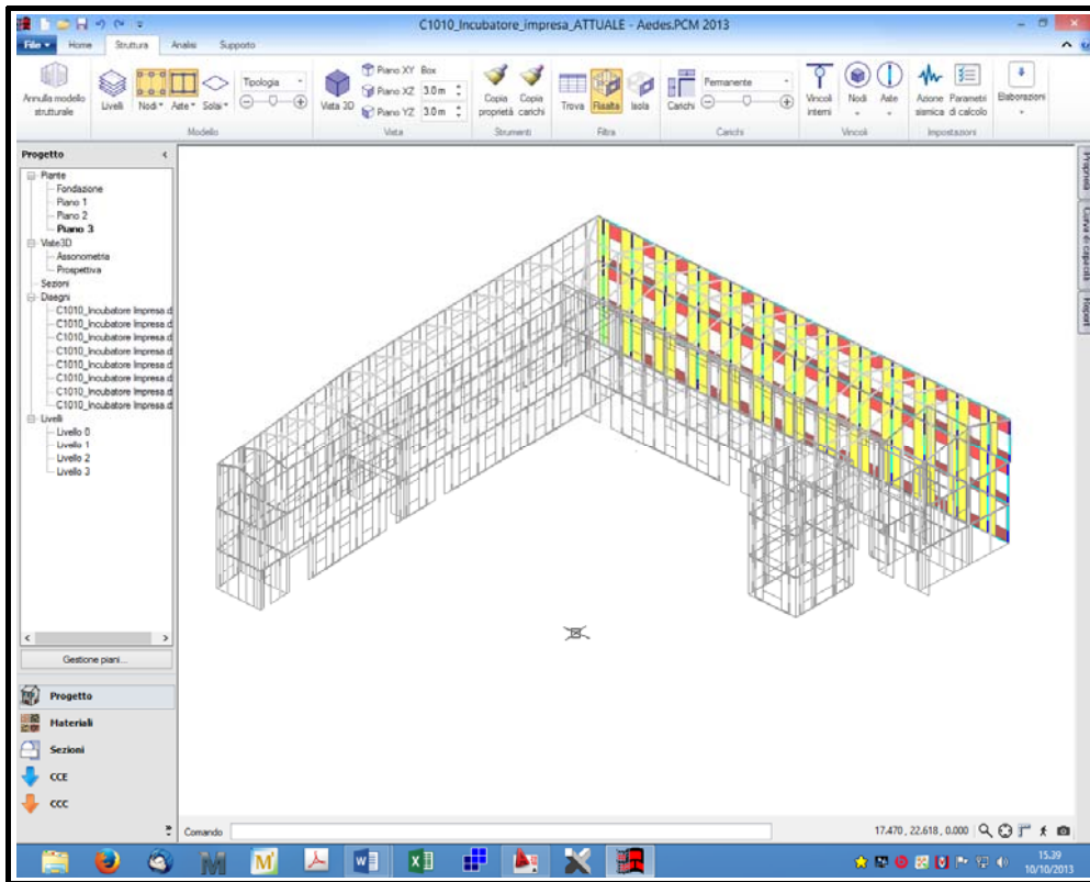
Figura 17– Paramento “B”
