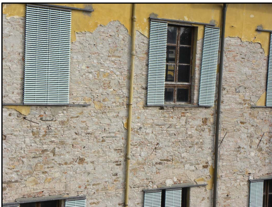
Figura 3 – Prospetto Sud- Particolare della tipologia di muratura
