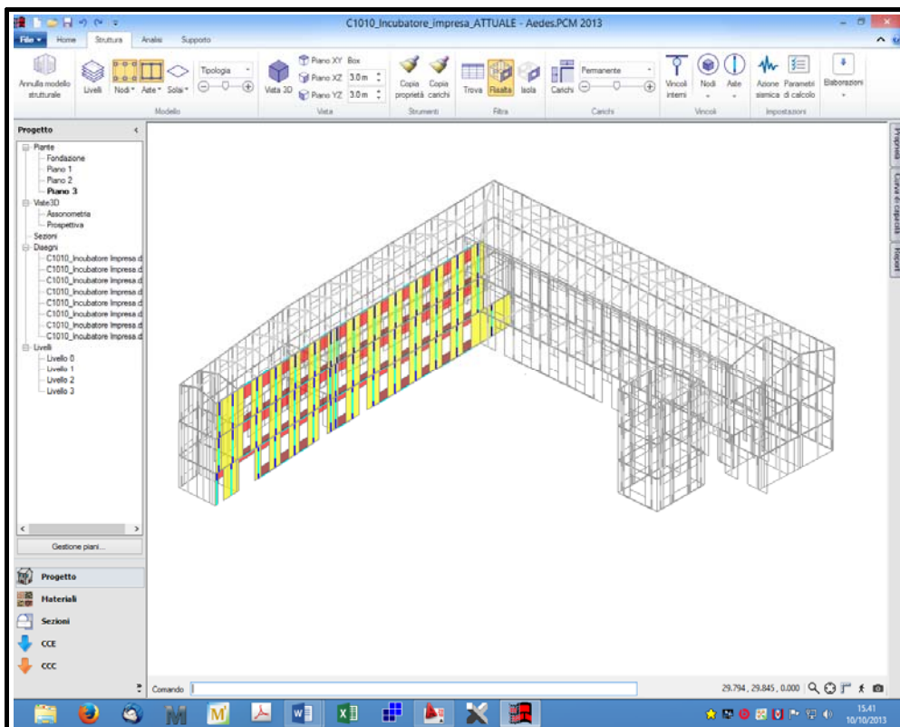
Figura 18– Paramento “C”
