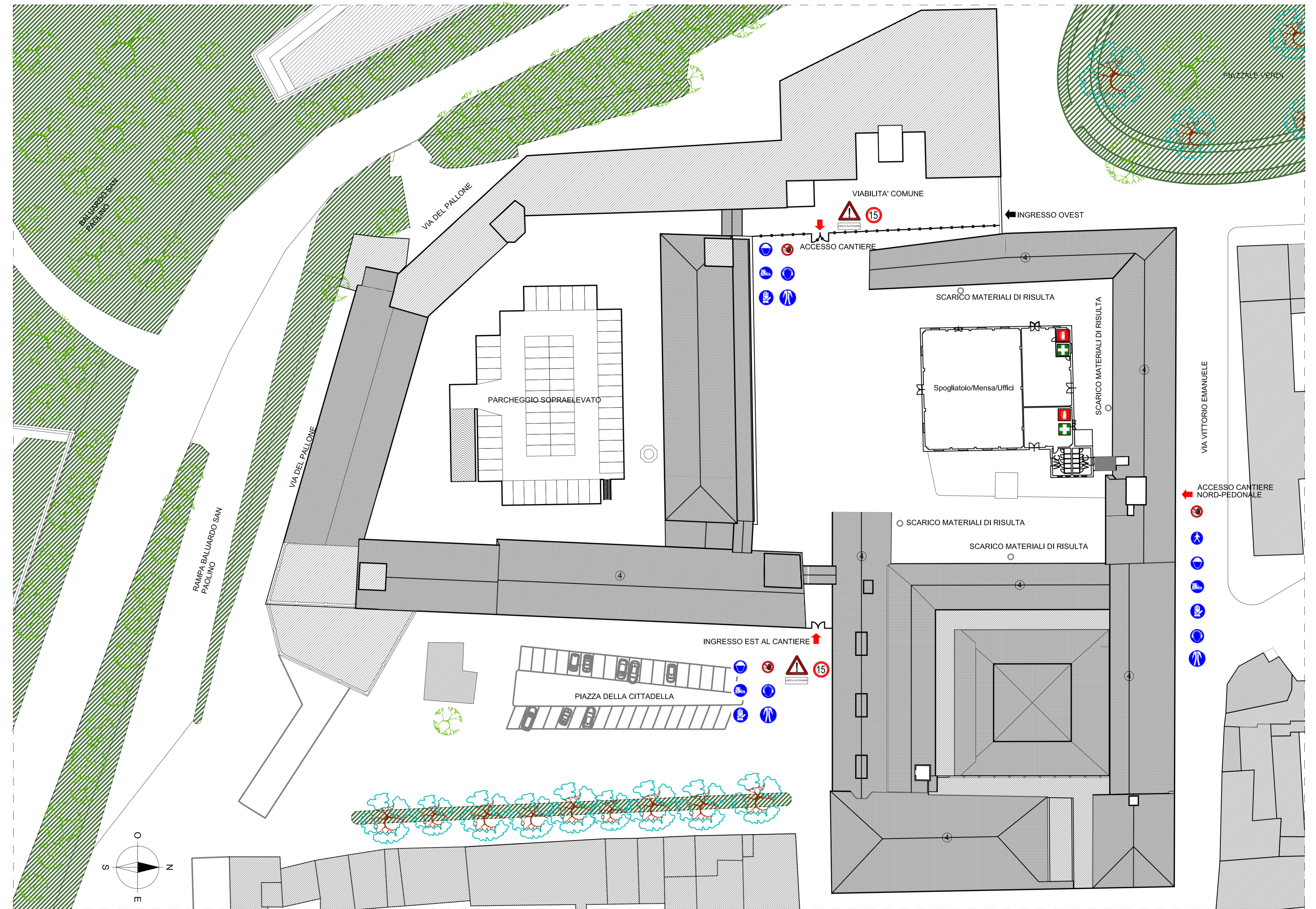
FASE 2 Demolizioni interne 1:500
