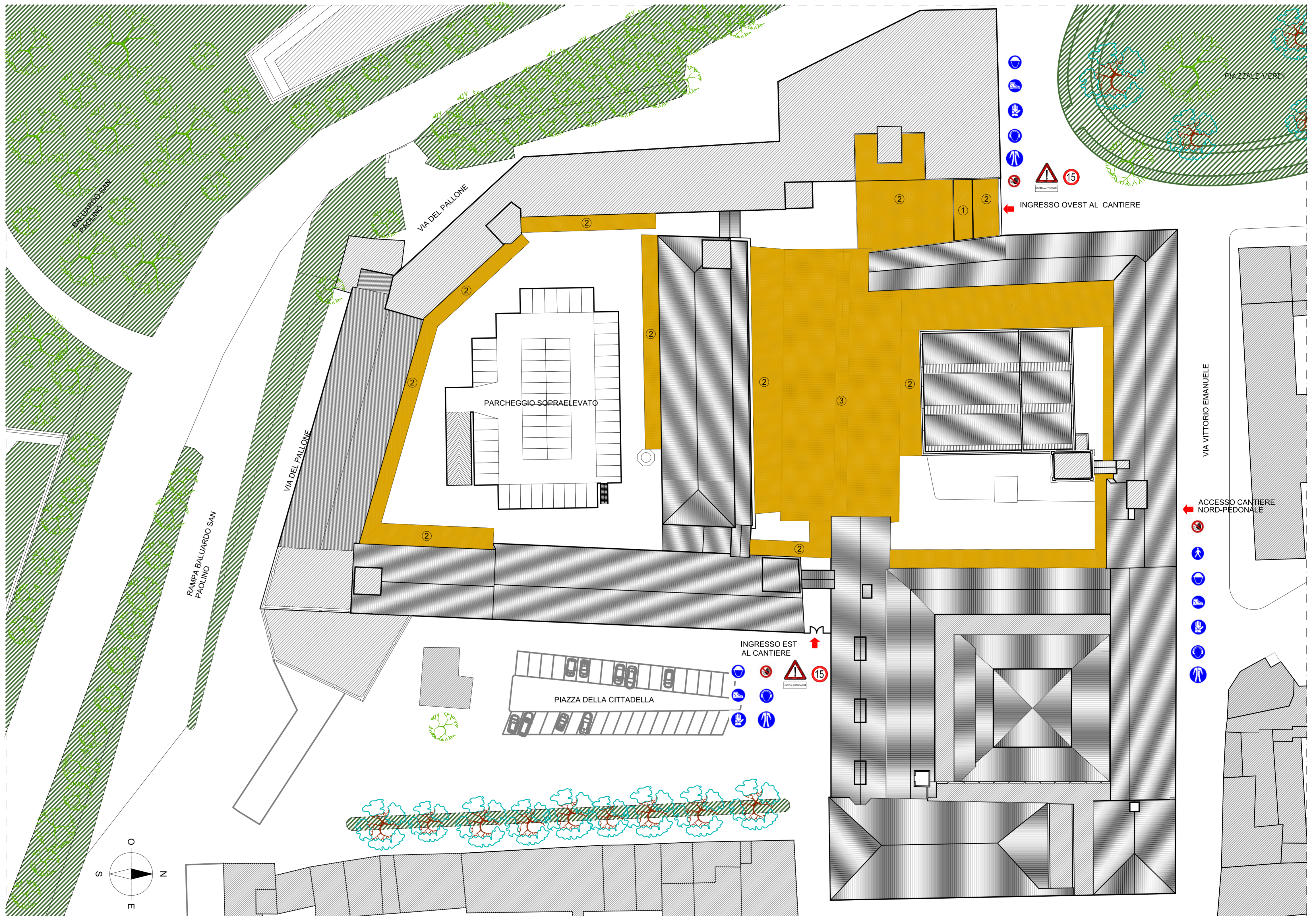
FASE 1 Demolizioni esterne 1:500
