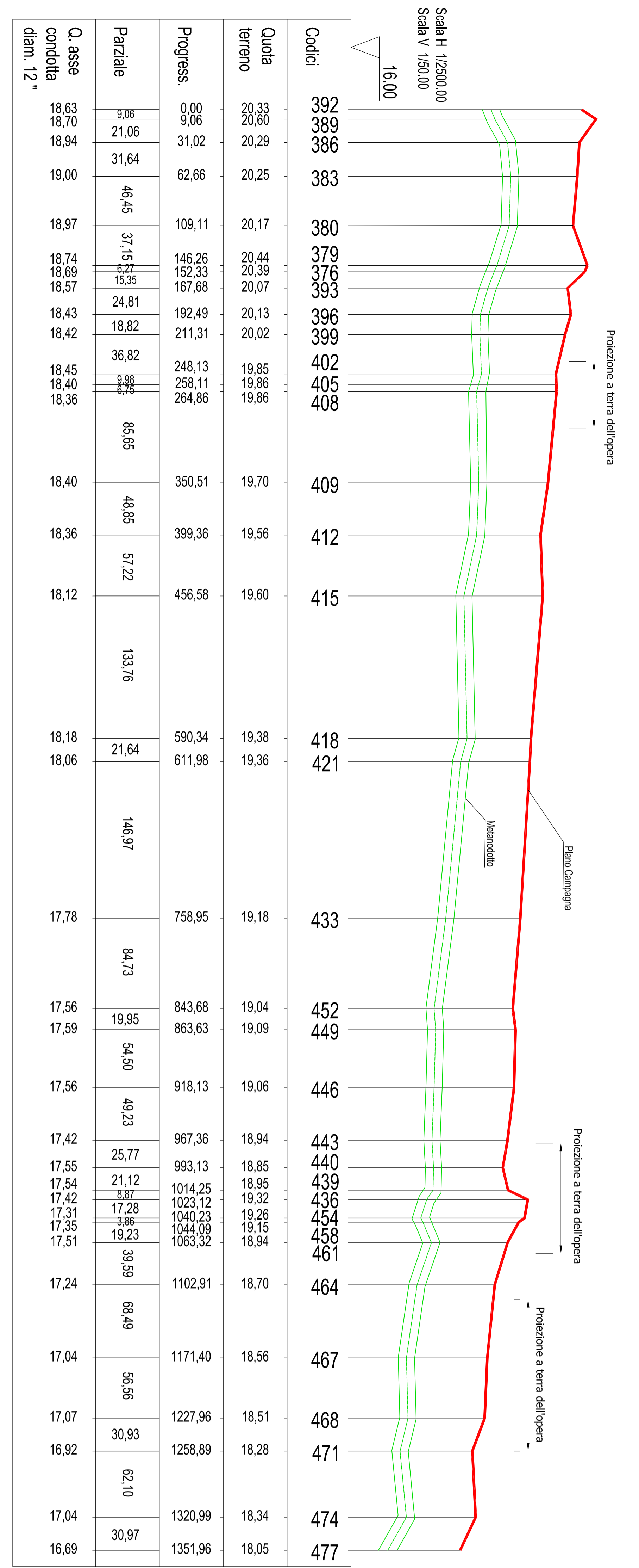
PROFILLO LONGITUDINALE CONDOTTA SNAM-002
