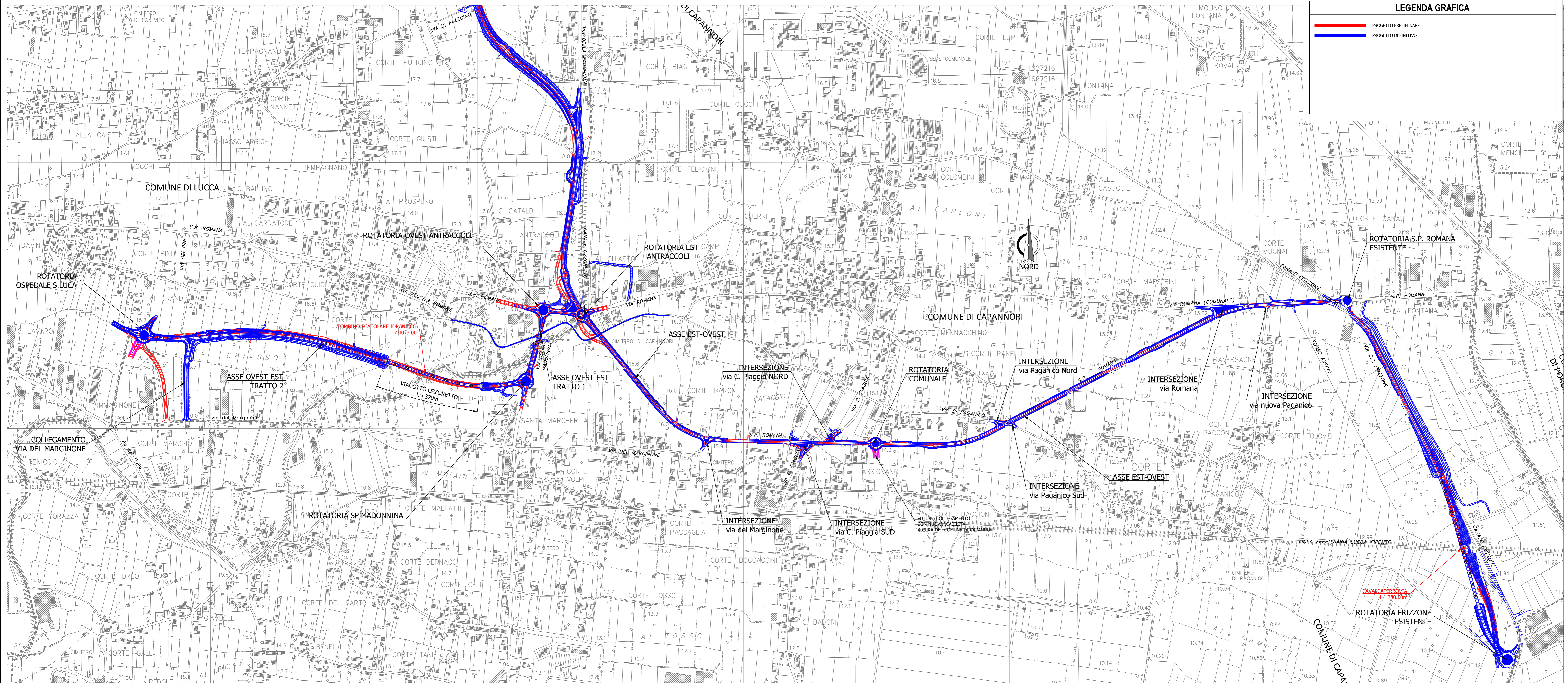
ASSI OVEST-EST E EST-OVEST SCALA 1:5.000
