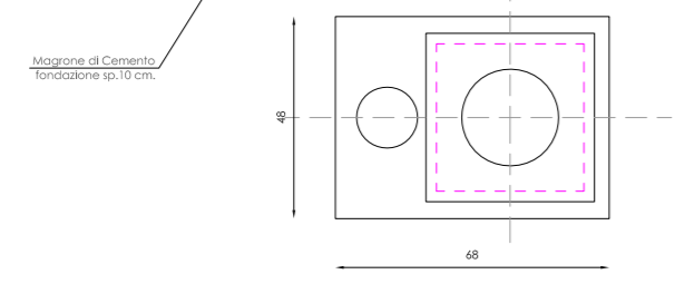
PARTICOLARE COSTRUTTIVO CAVIDOTTO INTERRATO - SU PORZIONE STRADALE
