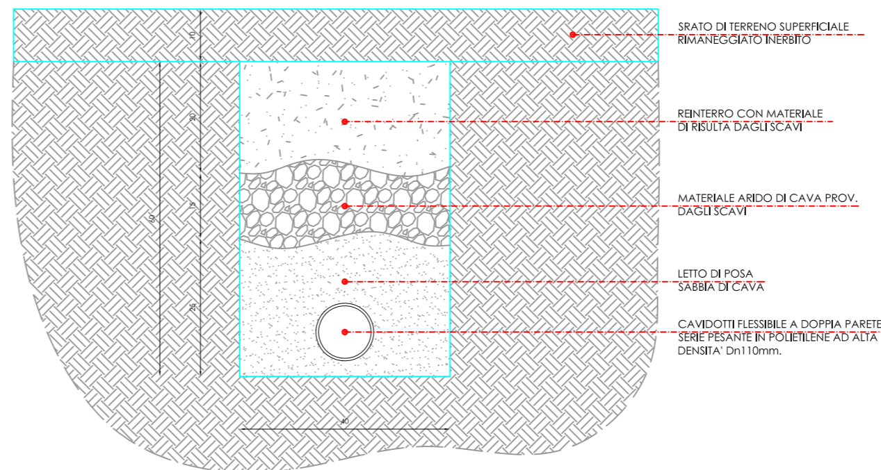
PARTICOLARE COSTRUTTIVO CAVIDOTTO INTERRATO - SU PORZIONE DI STERRATO E/O CUNETTA
