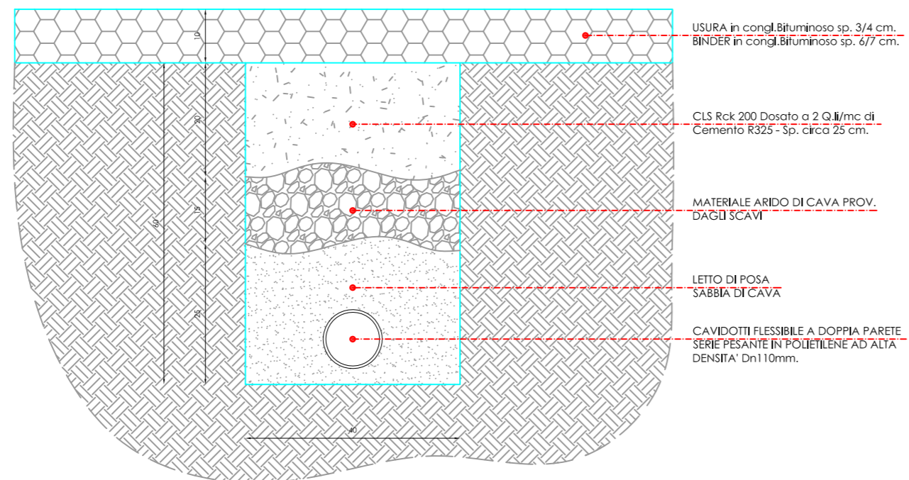
PARTICOLARE COSTRUTTIVO CAVIDOTTO INTERRATO - SU PORZIONE STRADALE
